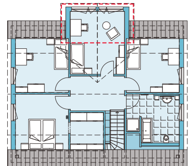
DACHGESCHOSS
