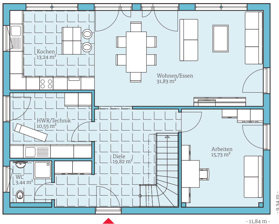
ERDGESCHOSS
